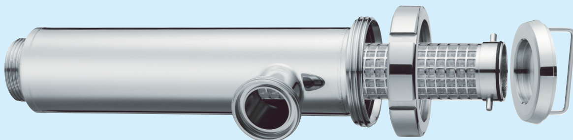
Eckrohrsieb mit Siebeinsatz in „Sandwichausführung“
